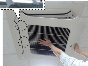
Einfügen der Kante in den Panelkörper
