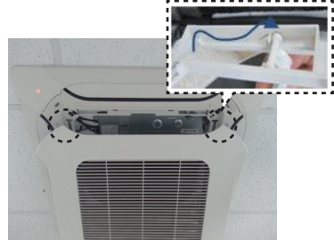
Einbauen der Rostverbindung am Bedienungsfeld
