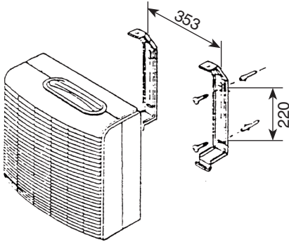
Bild 6: Maße für die Wandbefestigung
