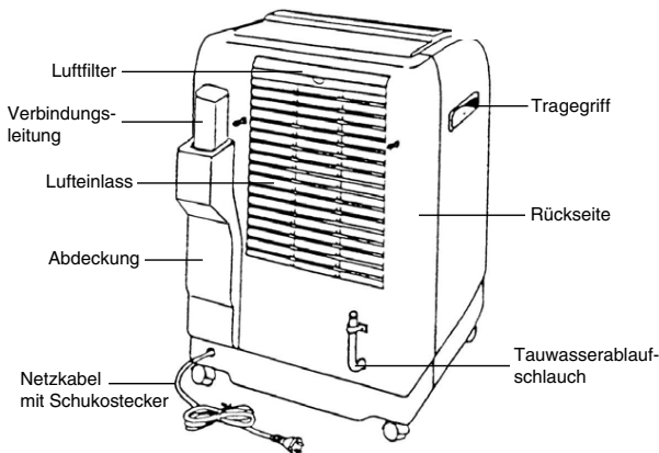
Bild 1: Aufbau des Gerätes
