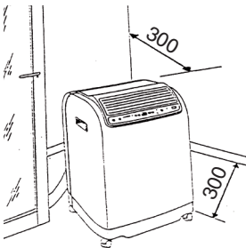
Bild 4: Aufstellung Innengerät
