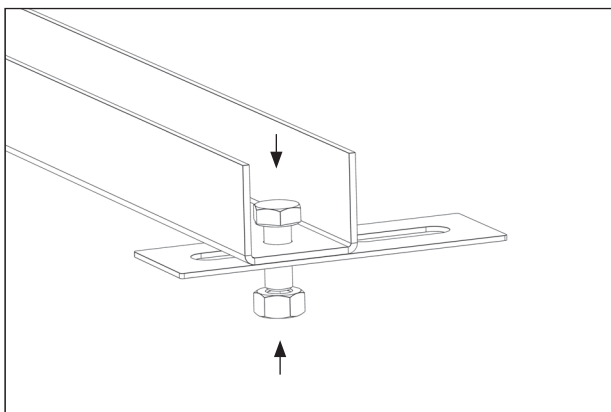
Montagehilfe + Montageschiene
