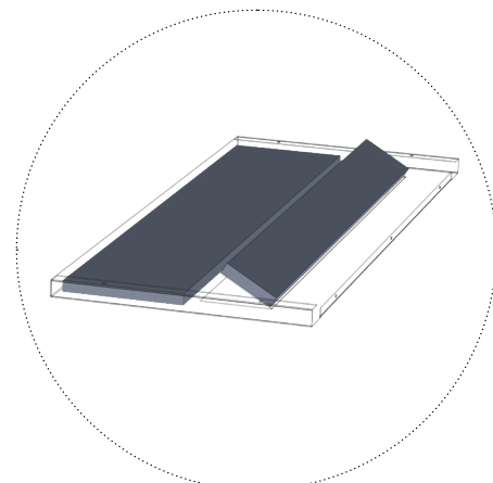
Einkleben des Schallschutzes mittig
